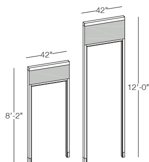
Steel Transom Door Frame
