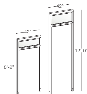
Glass Transom Door Frame
